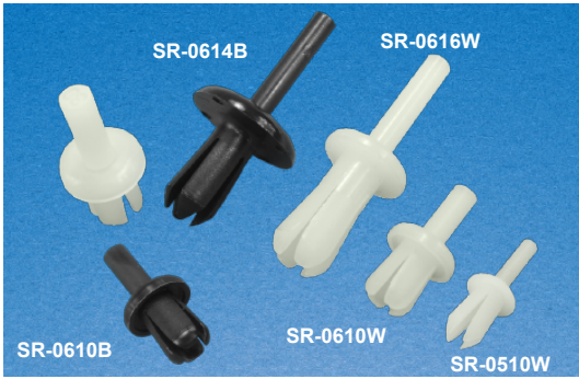
线槽或导轨专用铆钉
